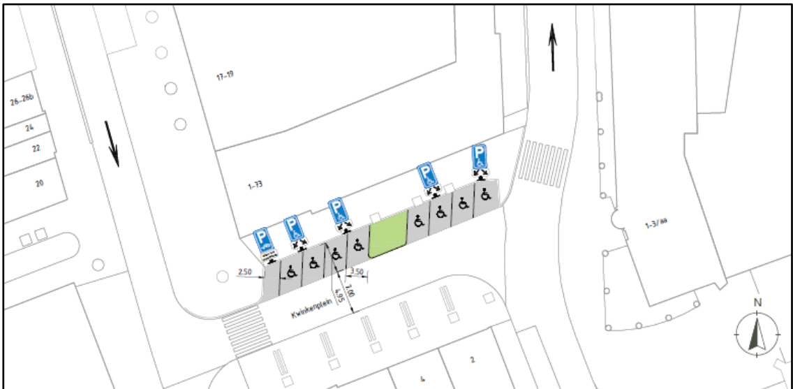
Ontwerp voor 8 ruime gehandicaptenparkeerplaatsen en plantenbakken (groene vlak) op het Kwinkenplein. Helemaal links komt de deelautoparkeerplaats voor GreenWheels.
