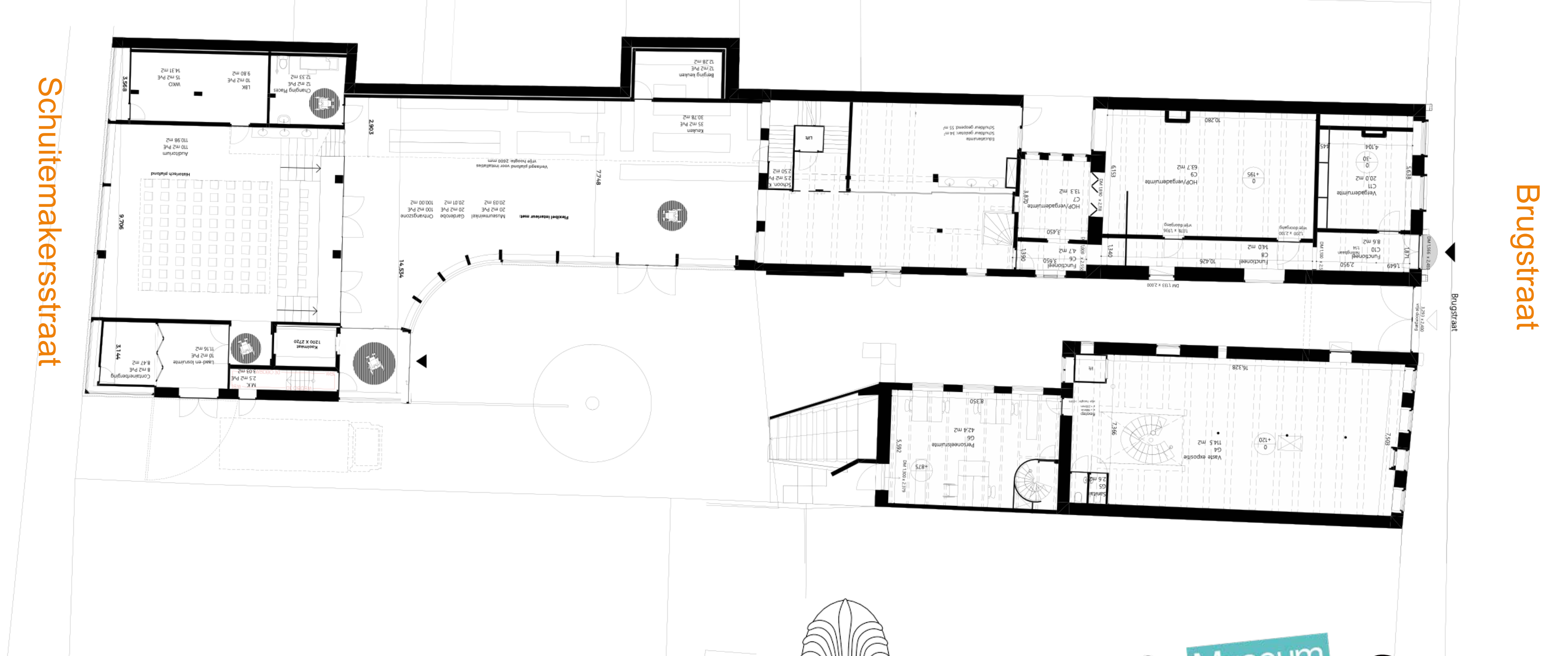
Begane grond
